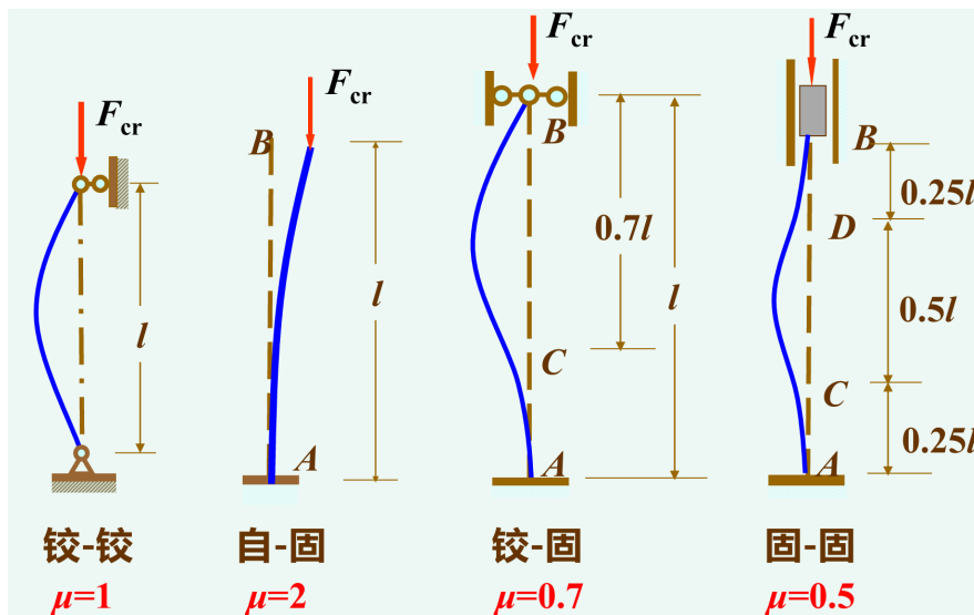
图 24: 不同端部约束下压杆屈曲形态示意
