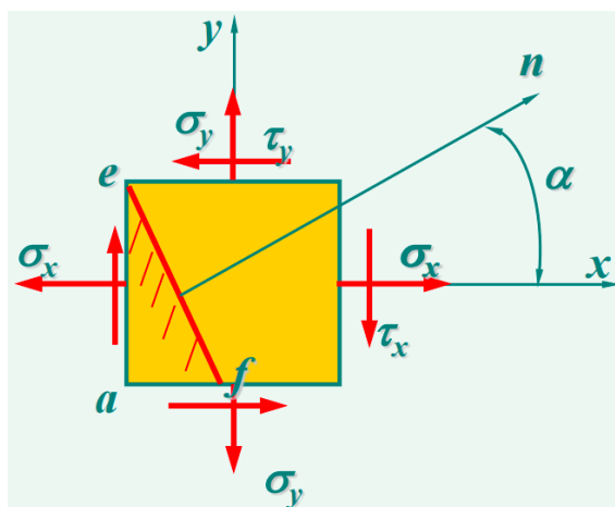
图 20: 平面应力状态与斜截面外法线
