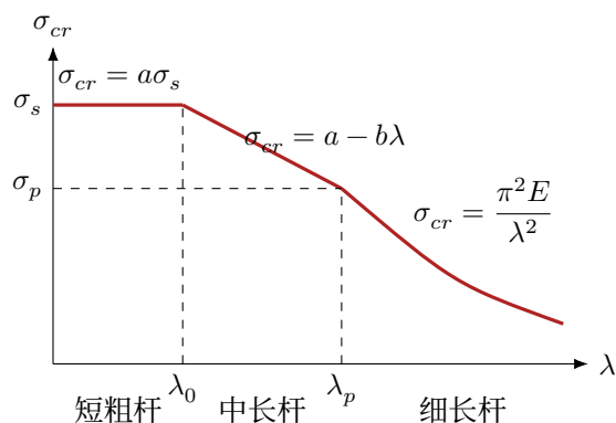
图 25: 临界应力总图
