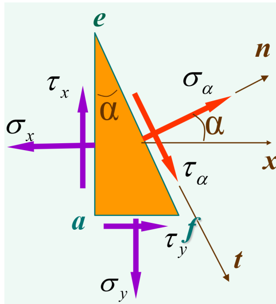
图 21: 斜截面上应力
